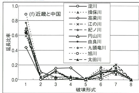
堤防被災形式の「近畿と中国」地方整備局河川による違い (中間的な照査評価)
